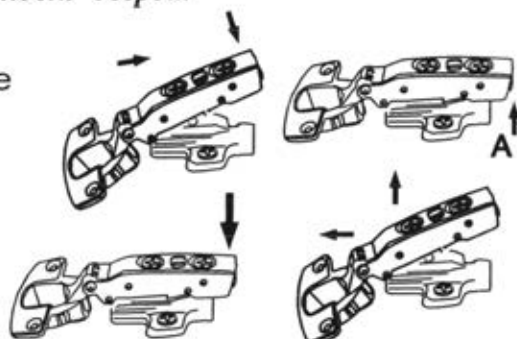
Схема монтажа петли.
